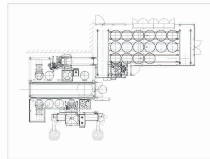
■ Schéma de la ligne de pétrissage linéaire
